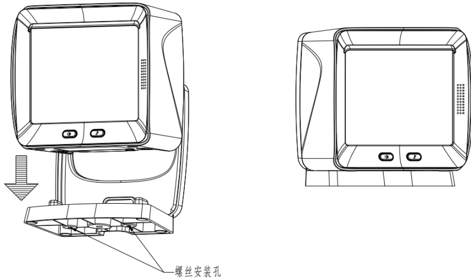
图 2-3 底座装配示意图
