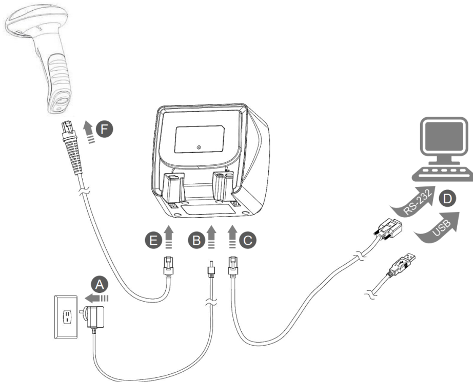
图 3-3 线缆连接示意图
