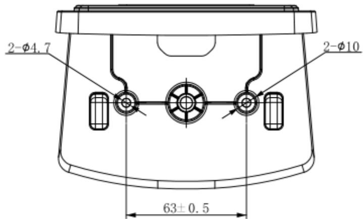
图 2-4 底座固定点尺寸图
